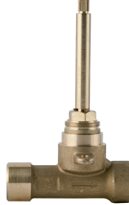
Cuerpo llave de paso -izda. -1/2" In wall Shut off valve -left-1/2" 016237.0AR.99
